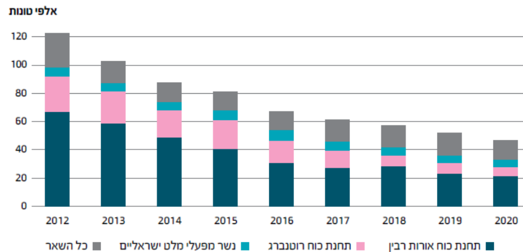
איור 11 פליטה לאוויר של תחמוצות חנקן במפל"ס, אלפי טונות
