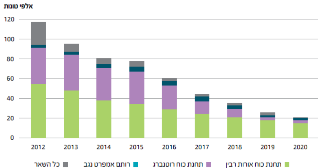
איור 14 פליטה לאוויר של תחמוצות גופרית במפל"ס, אלפי טונות
